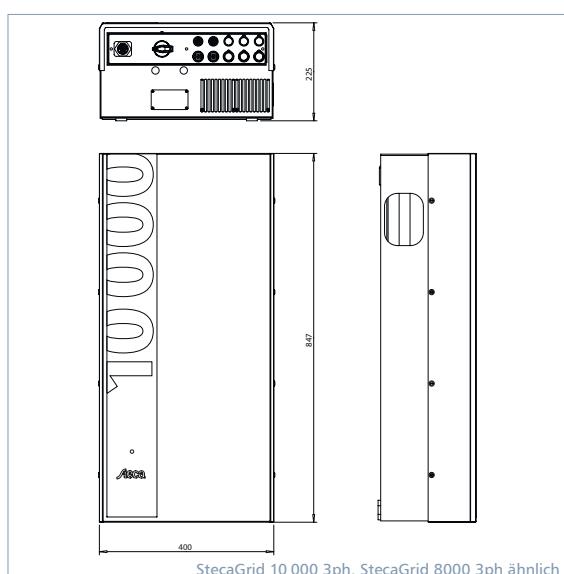
StecaGrid 10 000 3ph, StecaGrid 8000 3ph ähnlich
